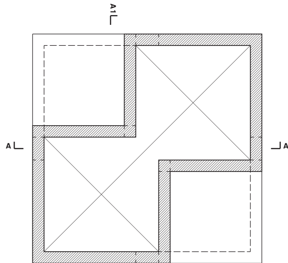
Grundriss +6,00
